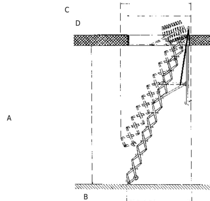
Tværsnit af Columbus lofttrappe. Rumhøjde (A), udledning (B), udklappning (C) og hulmålt (D).
