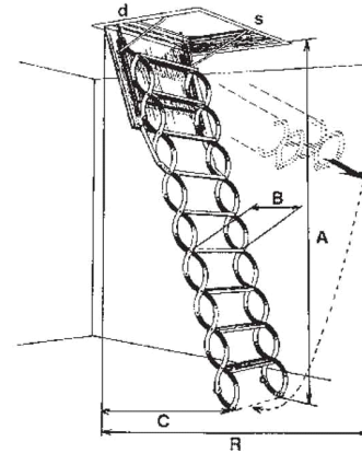
Principtegning af Lusso PP
