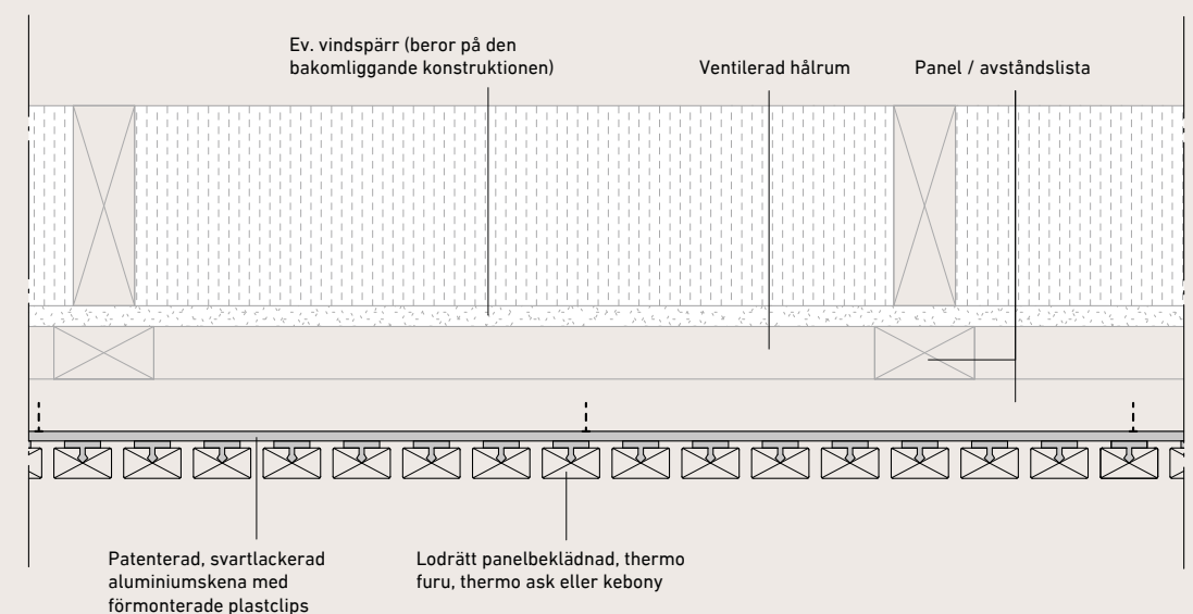
Lodrätt fasadbeklädnad
